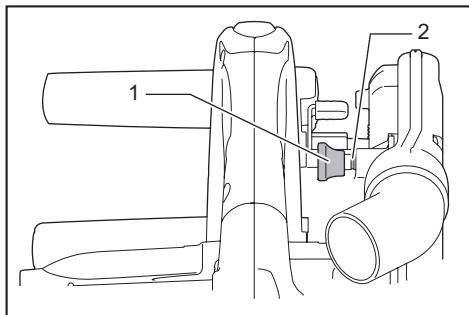
► 1. Butée 2. Marque rouge
