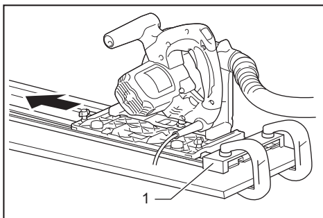
► 1. Fixed stop
