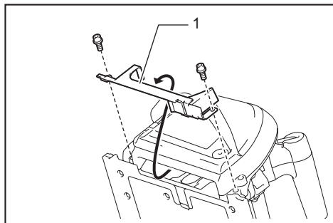
► 1. Collerette
