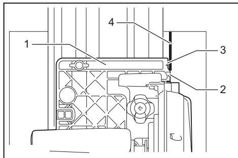
► 1. Base 2. Marca triangular externa 3. Marca triangular interna 4. Línea de corte
