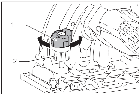
► 1. Freno rápido 2. Perilla de ajuste de profundidad
