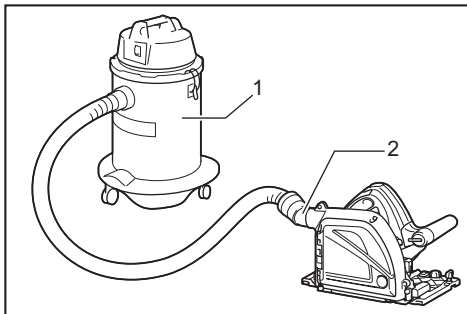
► 1. Aspirateur 2. Sortie de poussière
