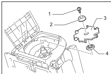
► 1. Perno hexagonal 2. Brida exterior 3. Disco de la ranuradora 4. Brida interior
