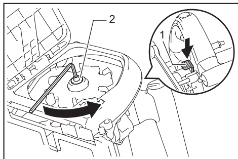
► 1. Bloqueo del eje 2. Perno hexagonal
